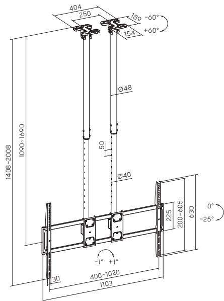
PLB-CE15610L
